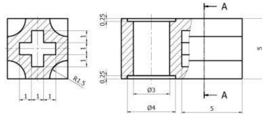
Corte A-A
