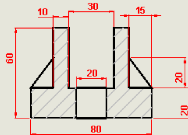
Corte Total A-A
